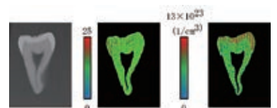
▲現在開発中の半導体型検出器を用いたエックス線撮影により、物質の実効原子番号や電子密度が分かります。単純X線画像(左)、実効原子番号のカラー画像(中央)、電子密度のカラー画像(右)。
